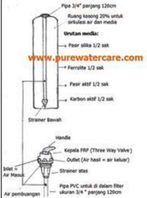
Cara Pemasangan Filter Air FRP 1054 dan Kepala FRP (Three Way Valve)
